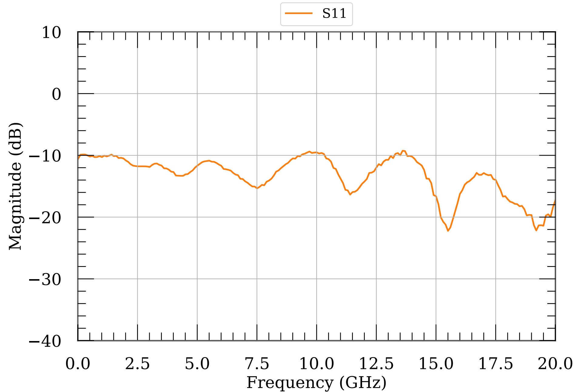
LNA S-params module019v2
